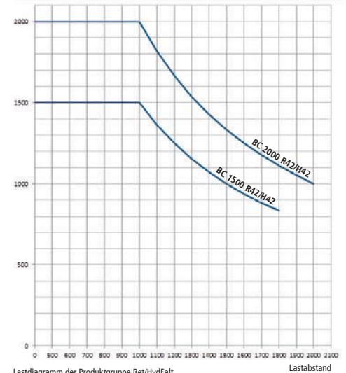
Lastdiagramm der Produktgruppe Ret/HydFalt
